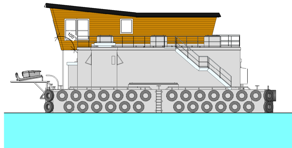
3 FASADE VELFERDSIDE 1 : 200
