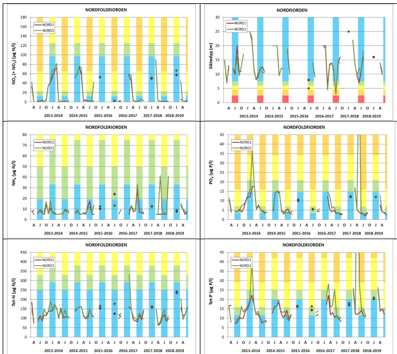
Figur 18. Tidsserie for parameterne nitrat, ammonium, total nitrogen, fosfat, total fosfor og siktdyp målt fra 2013 til 2019 i Nordfoldfjorden. Resultatene fra stasjon NORD1 (i rødt) og NORD2 (i grønt) er vist i samme tidsserie. Næringssaltene er midlet over 0 til 10 eller 15 m. Bokstavene J, A, J og O på x-aksen står for hhv. Januar, April, Juli og Oktober.
