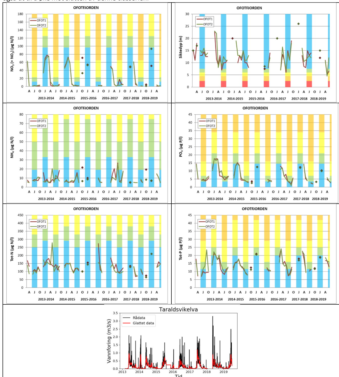
Figur 21. Tidsserie for parameterne nitrat, ammonium, total nitrogen, fosfat, total fosfor og siktdyp målt fra 2013 til 2019 i Ofothfjorden. Resultatene fra stasjon OFOT1 (i rødt) og OFOT2 (i grønt) er vist i samme tidsserie. Næringssaltene er midlet over 0 til 10 eller 15 m. Bokstavene J, A, J og O på x-aksen står for hhv. Januar, April, Juli og Oktober. Nederst er vannføringsdata fra Taraldsvikelva presentert.
