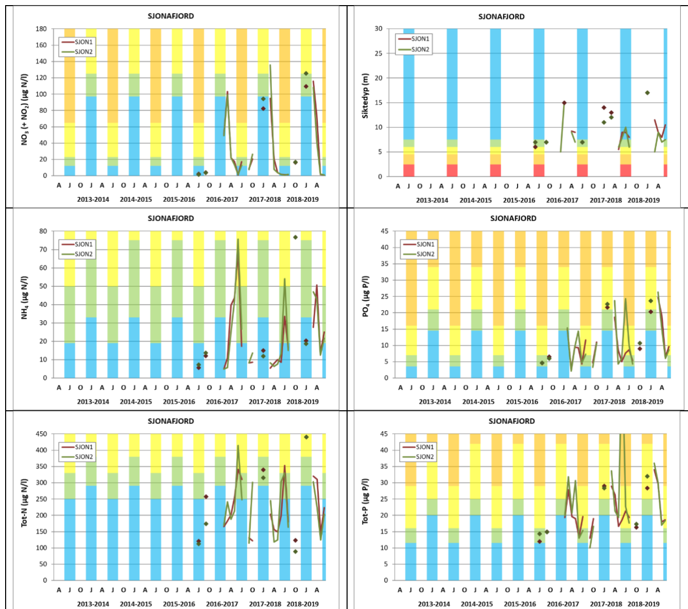
Figur 23. Tidsserie for parameterne nitrat, ammonium, total nitrogen, fosfat, total fosfor og siktdyp målt fra 2016 til 2019 i Sjona. Resultatene fra stasjon SJON1 (i rødt) og SJON2 (i grønt) er vist i samme tidsserie. Næringssaltene er midlet over 0 til 10 eller 15 m. Bokstavene J, A, J og O på x-aksen står for hhv. Januar, April, Juli og Oktober.
