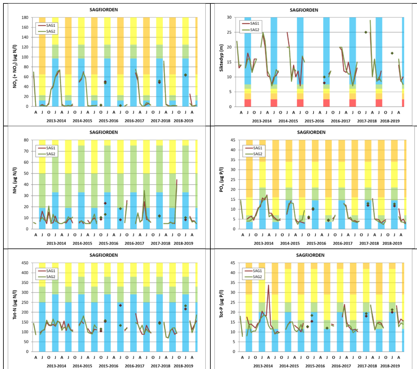
Figur 19. Tidsserie for parameterne nitrat, ammonium, total nitrogen, fosfat, total fosfor og siktdyp målt fra 2013 til 2019 i Sagfjorden. Resultatene fra stasjon SAG1 (i rødt) og SAG2 (i grønt) er vist i samme tidsserie. Næringssaltene er midlet over 0 til 10 eller 15 m. Bokstavene J, A, J og O på x-aksen står for hhv. Januar, April, Juli og Oktober.
